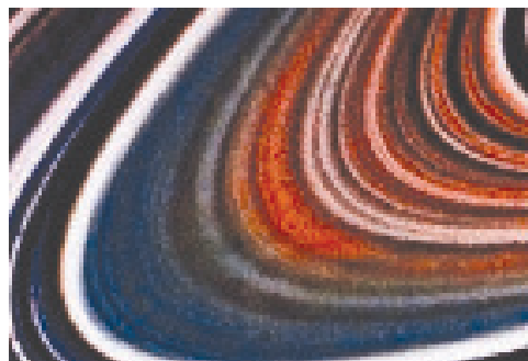
රූපය 7.18 - ඉලිප්සාකාර ගමන් මග
