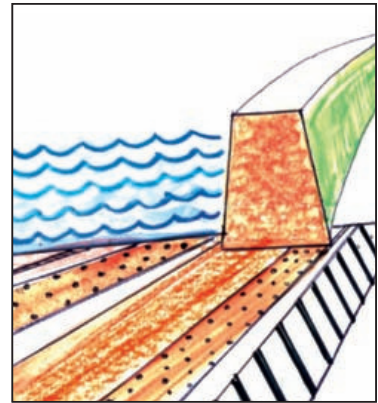
රූපය 4.3 - පාෂාණ ස්ථරවල ආනතිය
